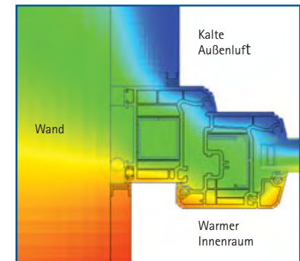
Waagerechter Querschnitt durch Fensterrahmen. Der Temperaturverlauf von -5 °C (blau) bis +20 °C (rot) macht deutlich, wie gut moderne Kunststofffenster dämmen.
