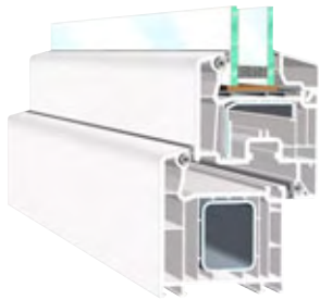
VEKA System SOFTLINE 70 AD flächenversetzt
