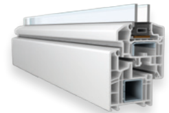
Flügelvariante halbflächenversetzt
